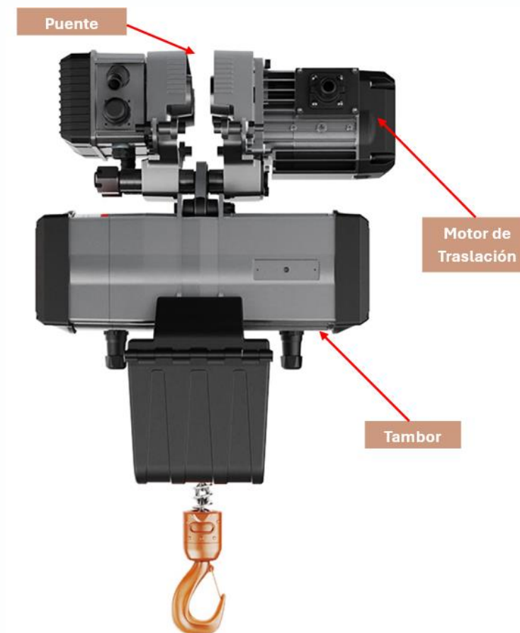
Figura N°2. Traslación del Puente
